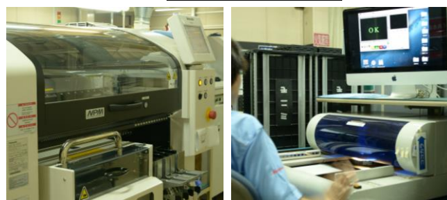
AOI 外観検査機
