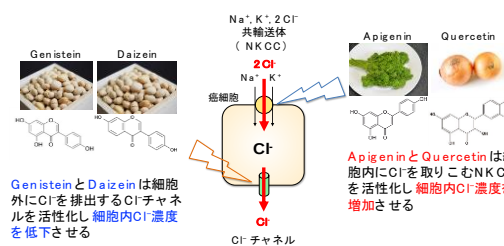
図3 フラボノイドによるCl - 輸送体・チャンネル活性制御
