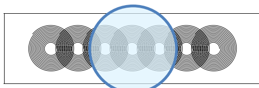
図1 円形平面コイルアレイと受電コイル
