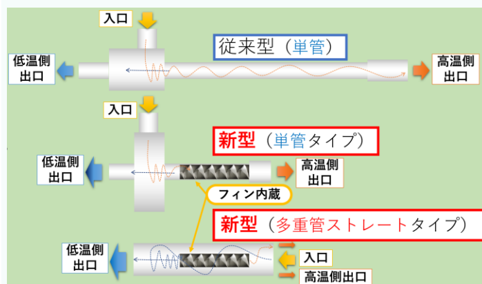
図1 螺旋状フィンを内蔵した新型ボルテックスチューブ
