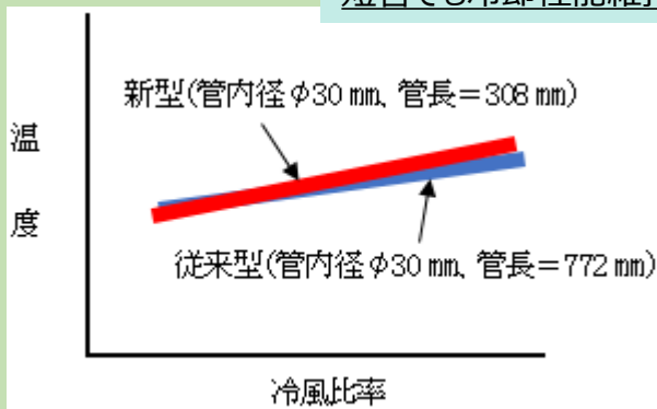
図3 長管と短管との冷却性能比較
