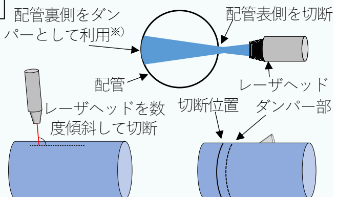
※) 配管裏側はレーザー光が広がることで切断されません
