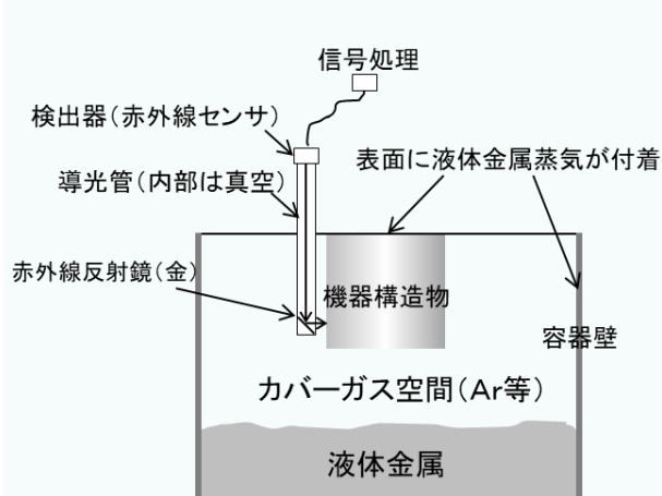
液体金属機器の金属蒸気付着モニター
