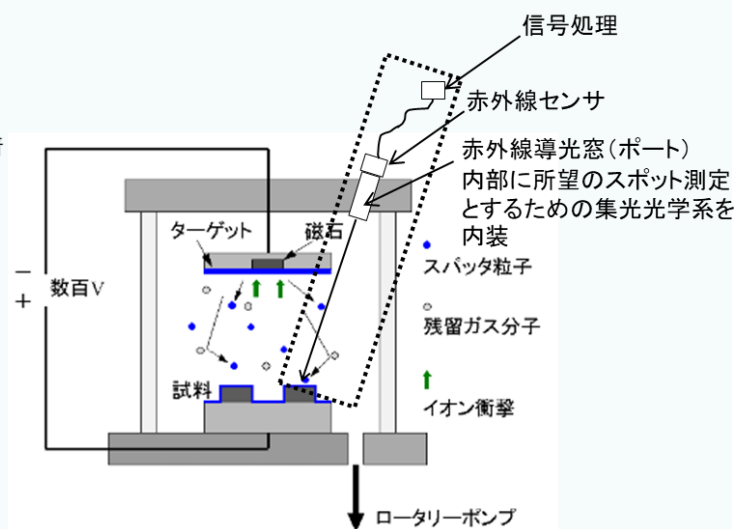
薄膜形成モニター
